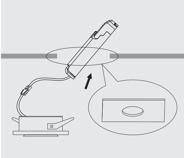
1. Ø53mm cutout
